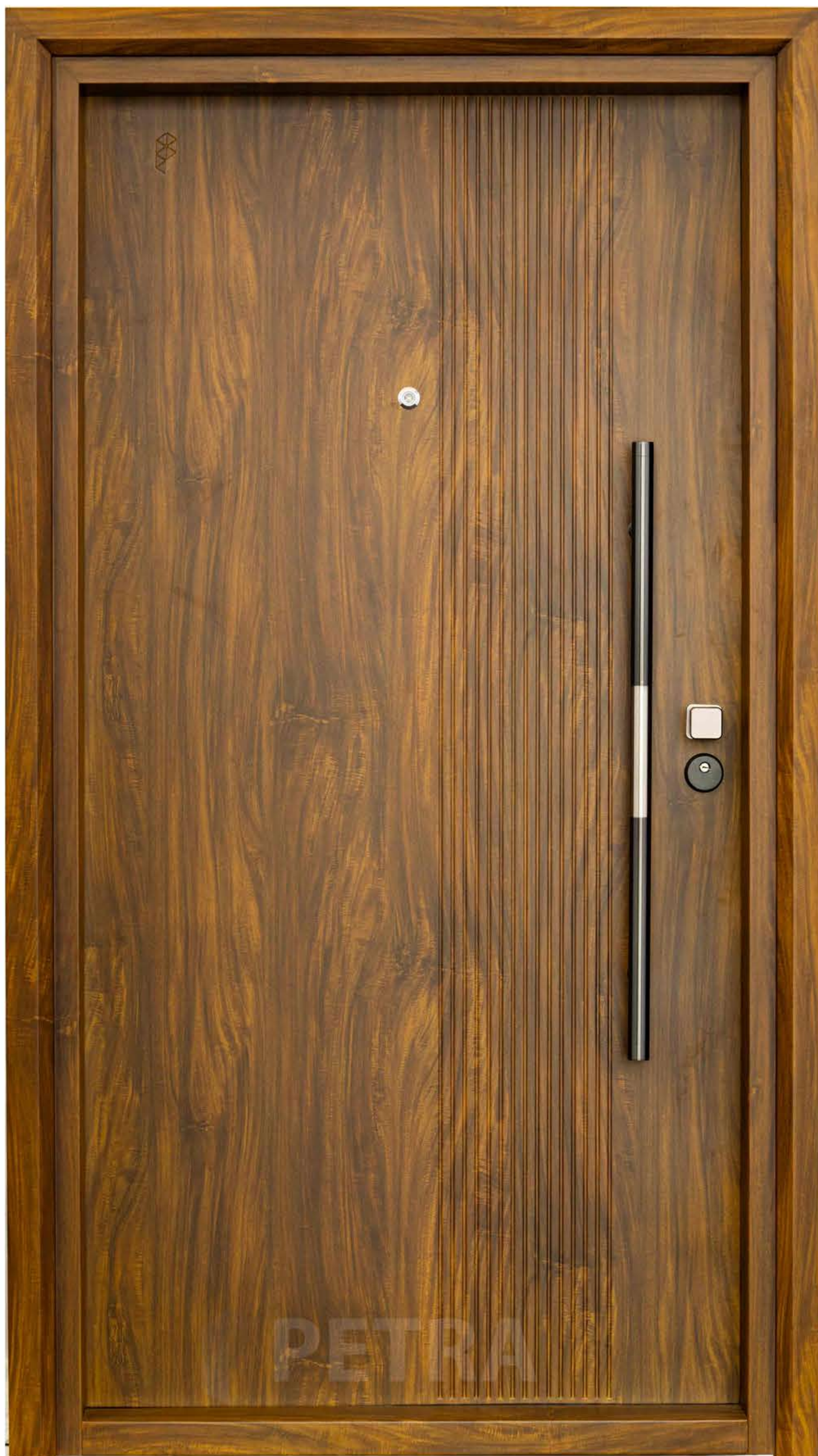
PTR 75 - 2050*1080*70MM 9" M/L (BH)
