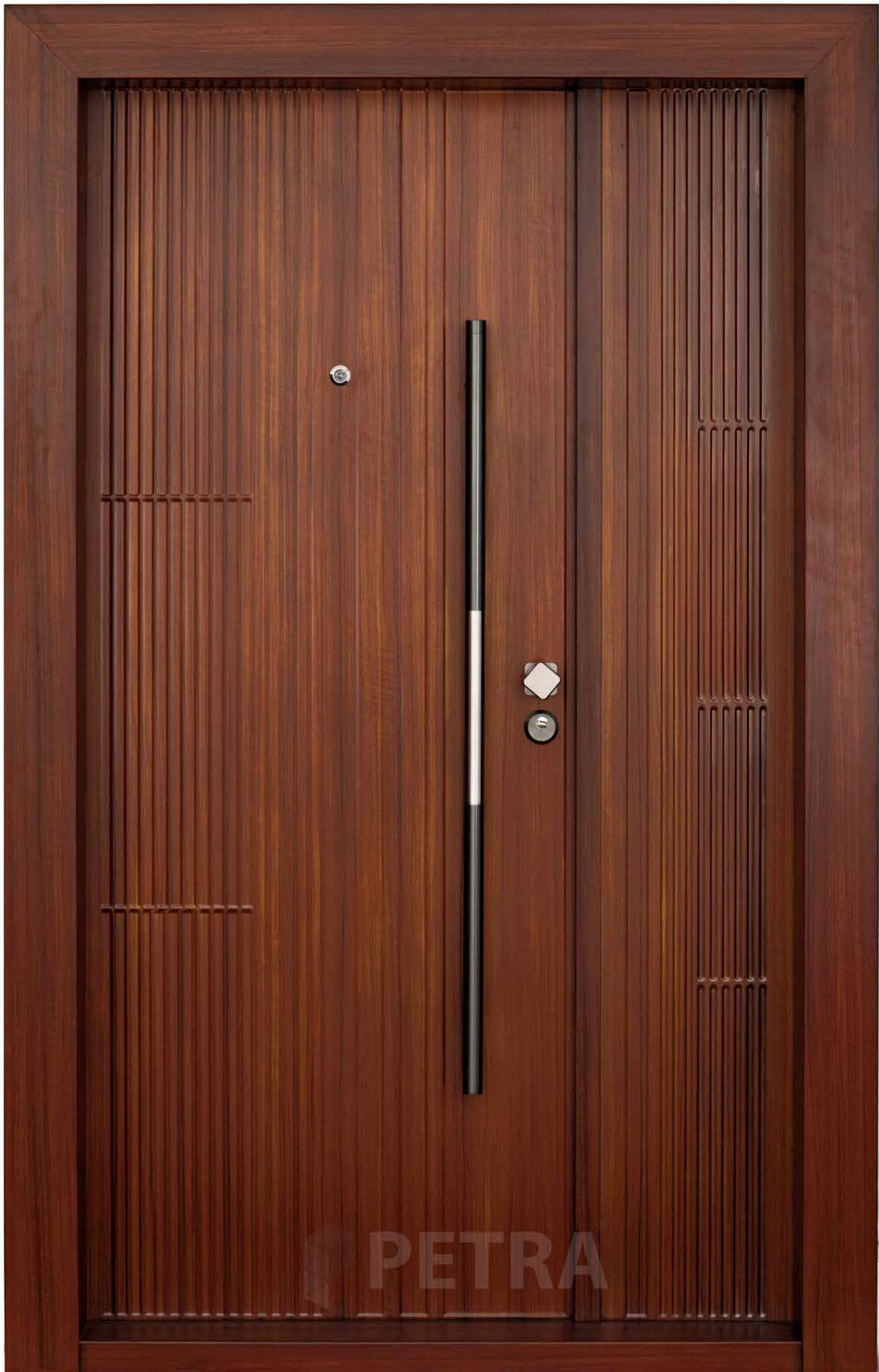
PTR 55 - 2050*1200*70MM 9" M\L MSBH
